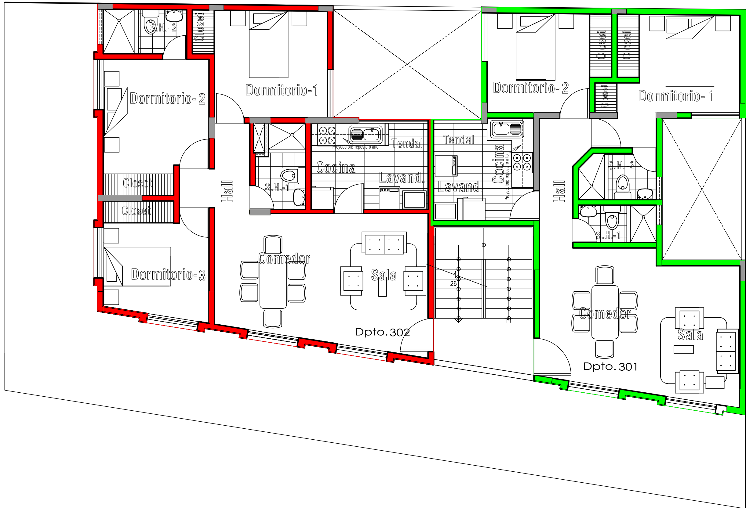
PLANTA: 3er PISO
